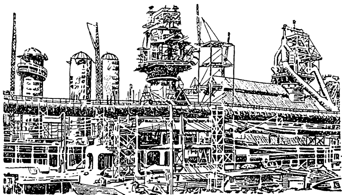
Общий вид доменного цеха Бузнецстроем
